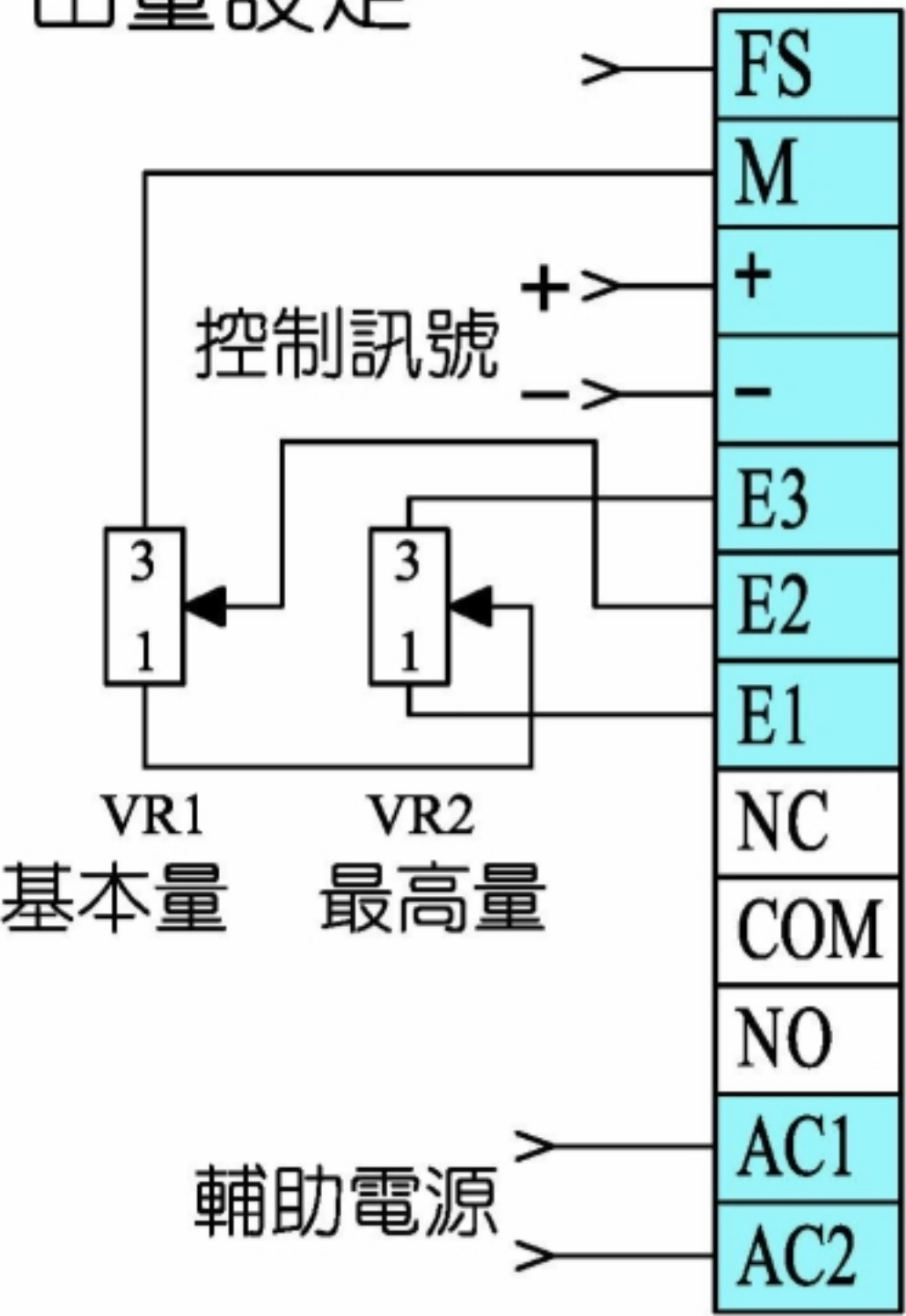
9. 基本輸出量及最高輸 出量設定
