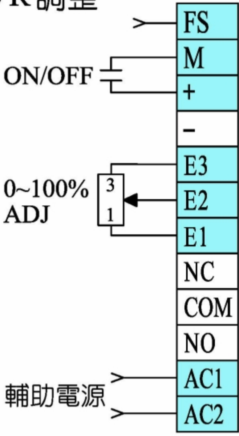
4. 乾接點訊號輸入，外 部 VR 調整
