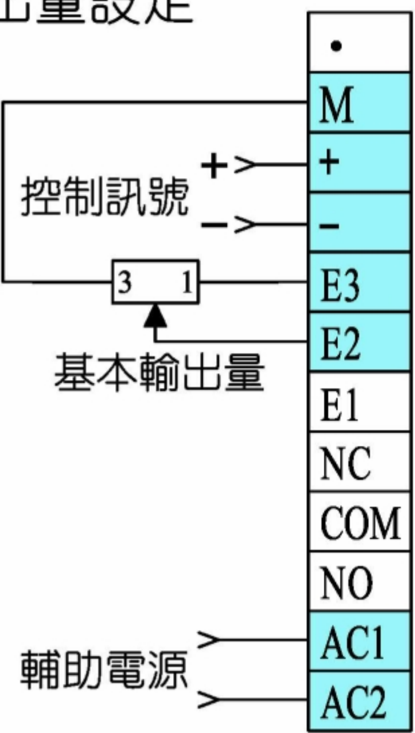
7. 控制訊號輸入，基本 輸出量設定
