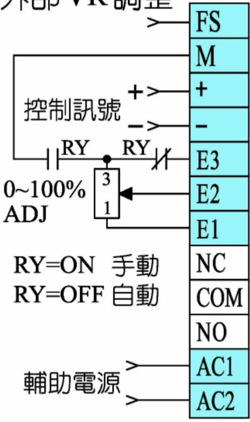
5. 手 - 自動 RELAY 切換 外部 VR 調整
