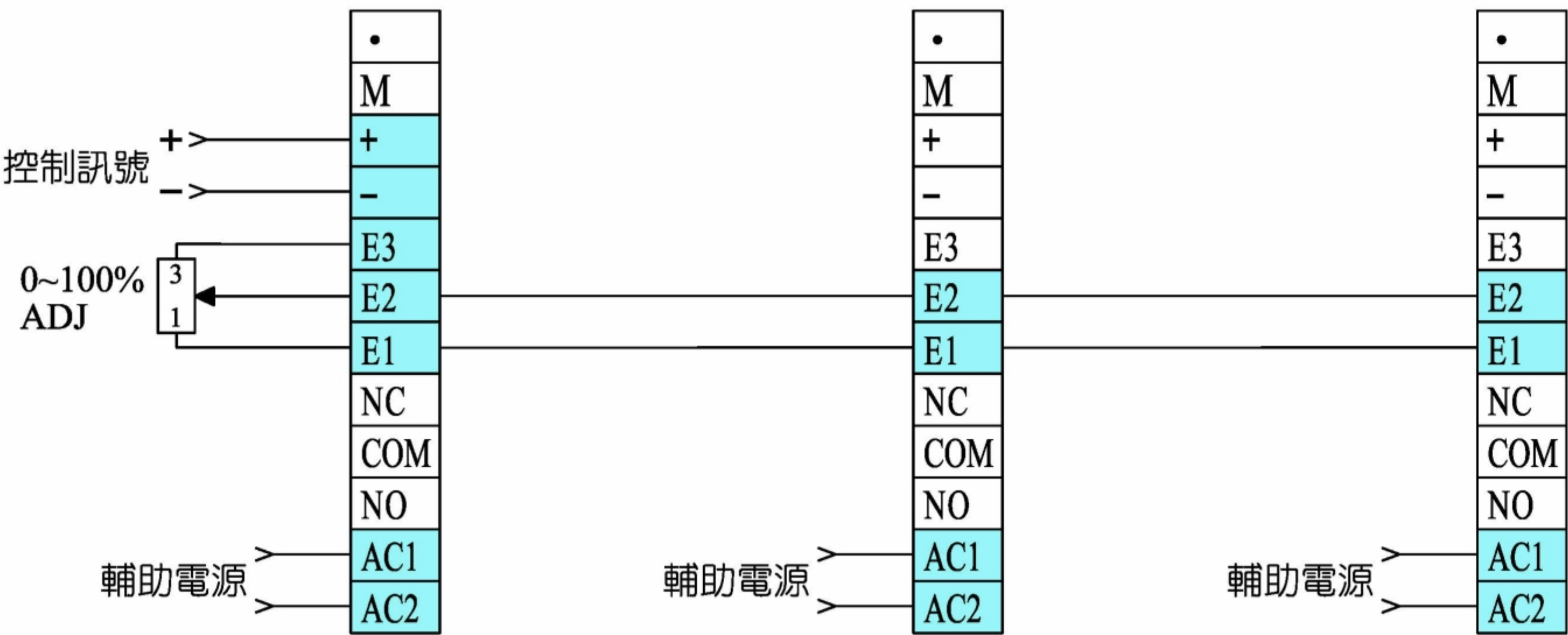
8. 多台連接，一只外部 VR 設定
