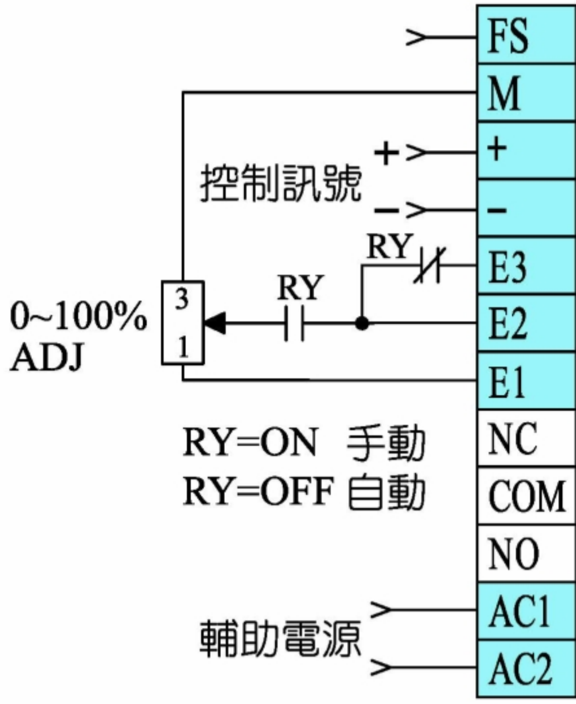
6. 手 - 自動 RELAY 切換
