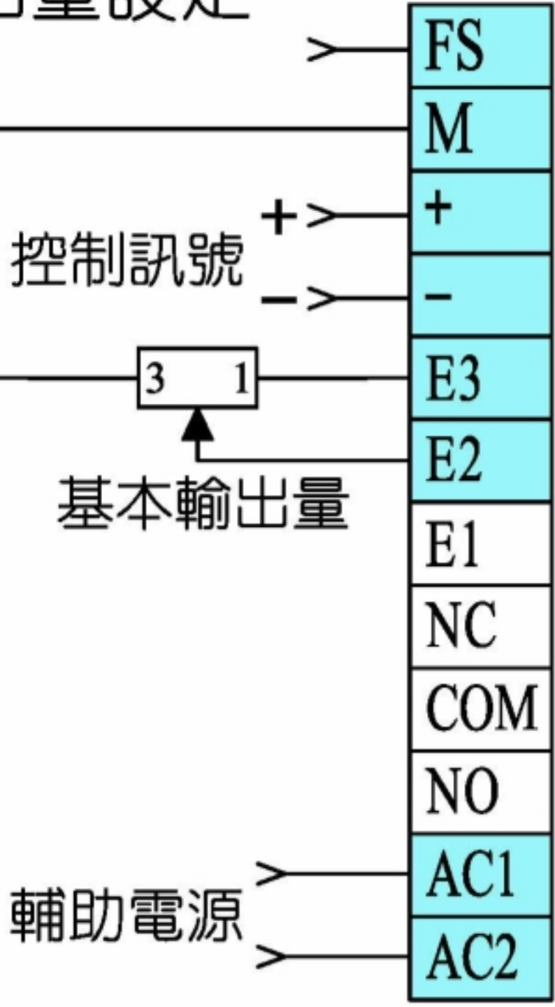
7. 控制訊號輸入，基本 輸出量設定
