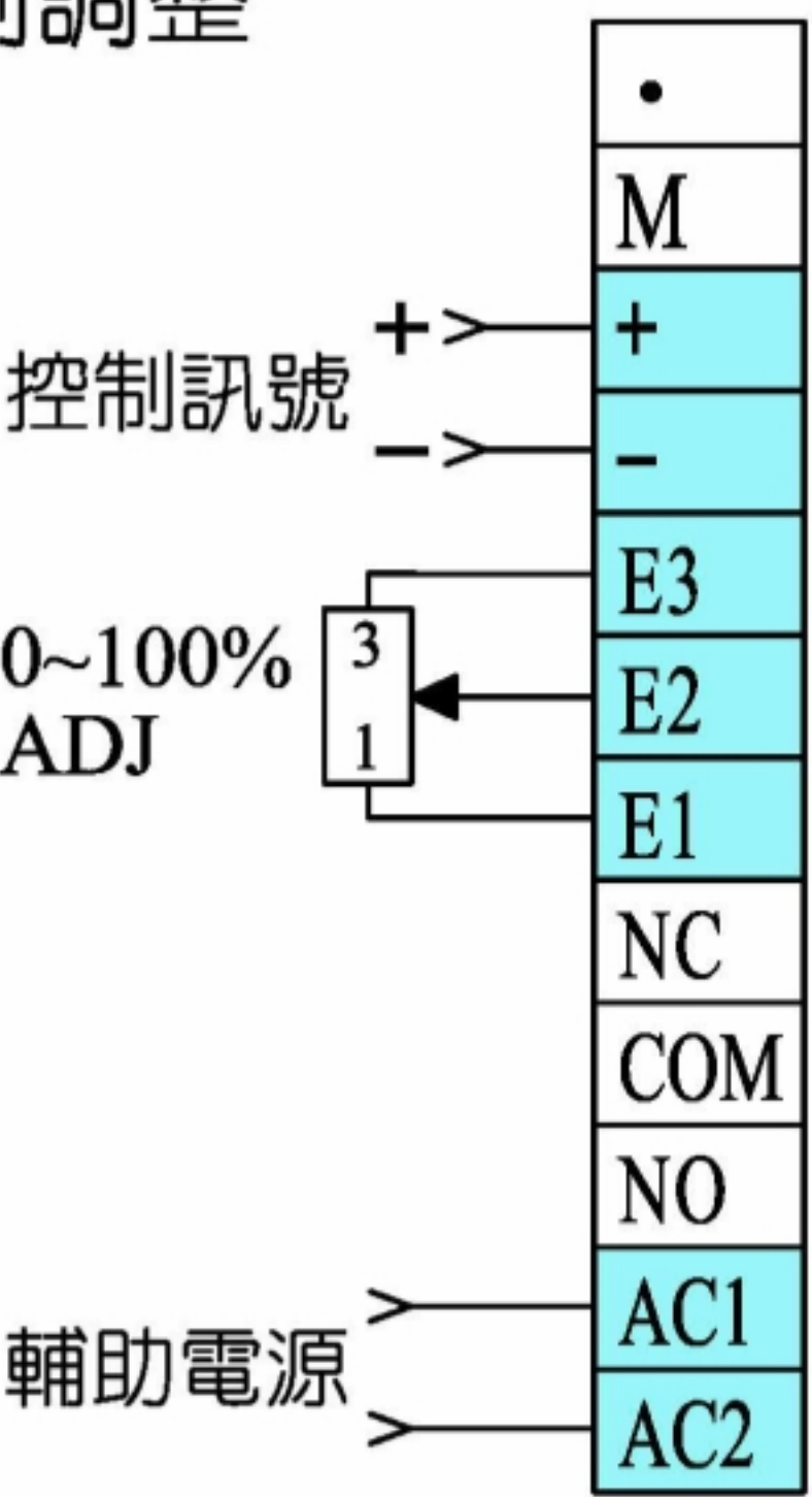
3. 控制訊號輸入，輸出 限制調整
