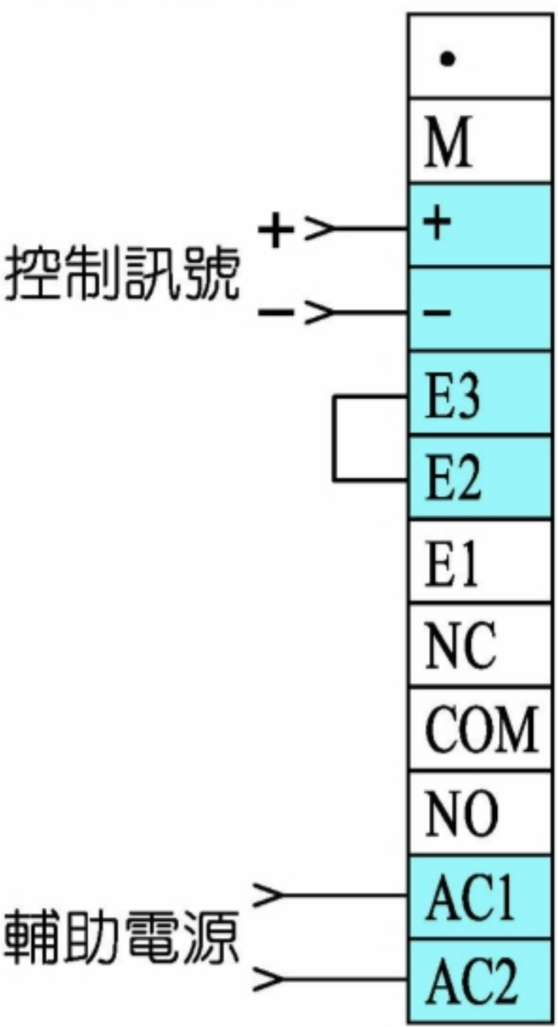
1. 控制訊號輸入
